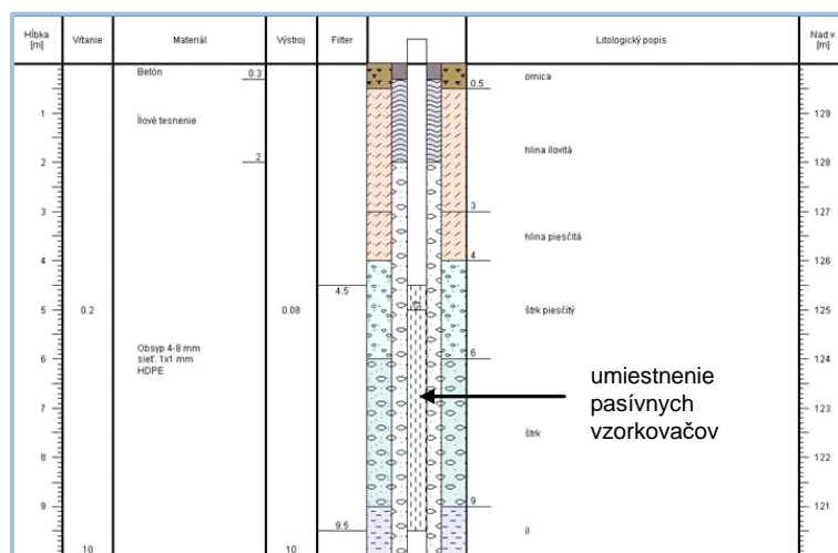
Obrázok 2.3.1.1. Skrátený projekt vrtu.
