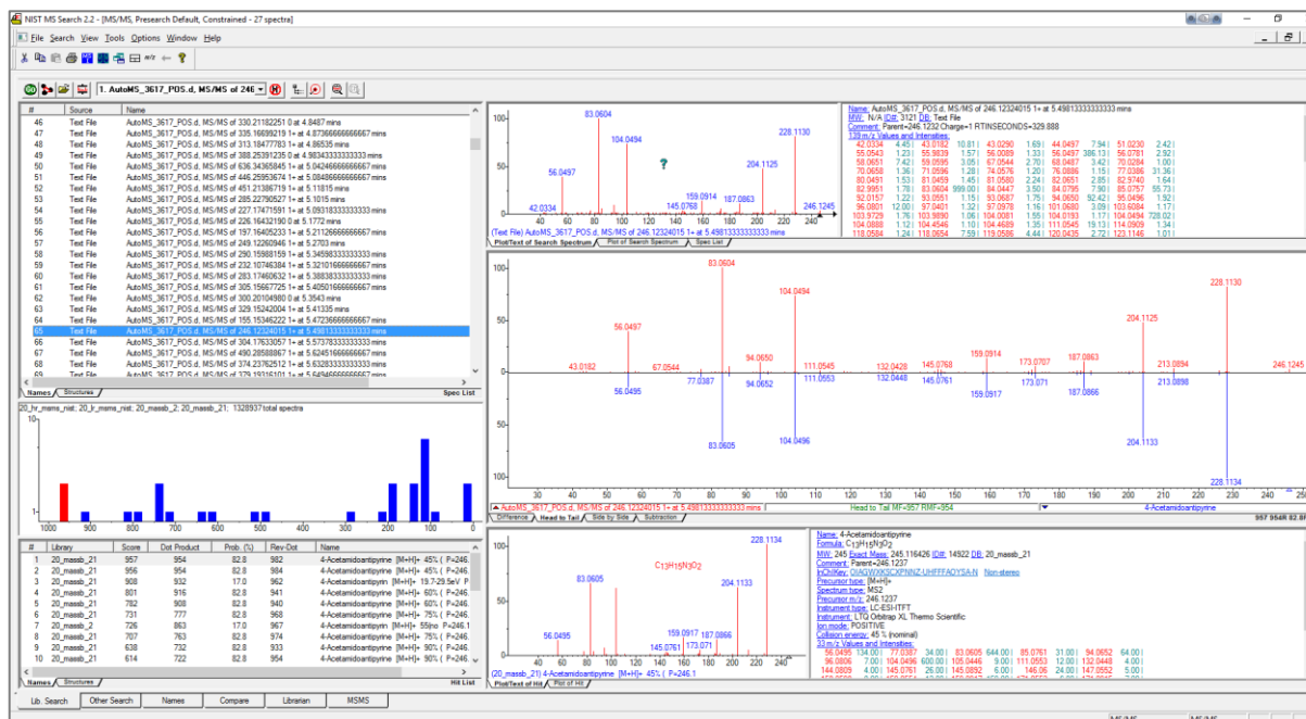
Obrázok 2.1.2.3.4. Identifikácia 4-acetamidoantipyrínu v prostredí NIST Search. Stredný panel pravo znázorňuje porovnanie experimentálneho (červené, hore) a knižničného MS/MS spektra (modré, dole) v zrkadlovom zobrazení.
